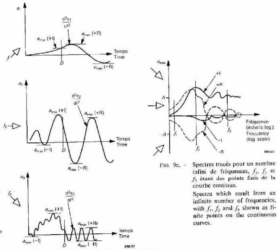
FIG. 9b. — Réponses pour les fréquences f_1 , f_2 et f_3 . Responses for f_1 , f_2 and f_3 .
