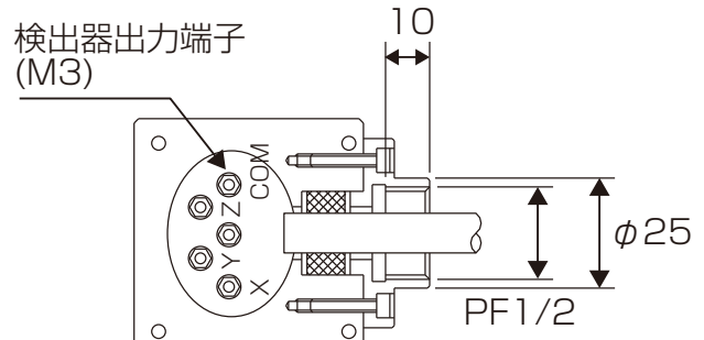
【イーイ断面】
