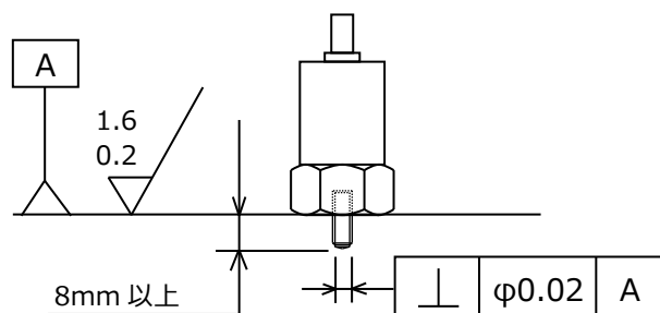
図4-2 ピックアップ取り付け面の加工
