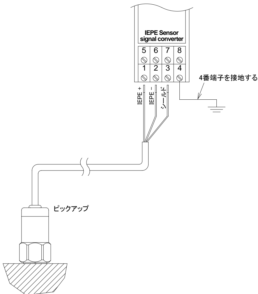
図 A-1 ピックアップが設置箇所が接地されていない場合の接地方法
