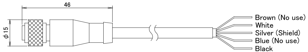
MS-AC010-5 ストレートコネクタ
