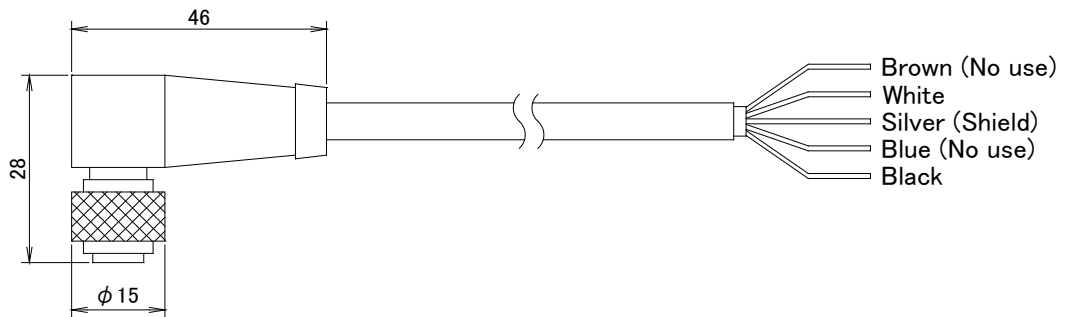
MS-AC011-5 ライトアングルコネクタ
