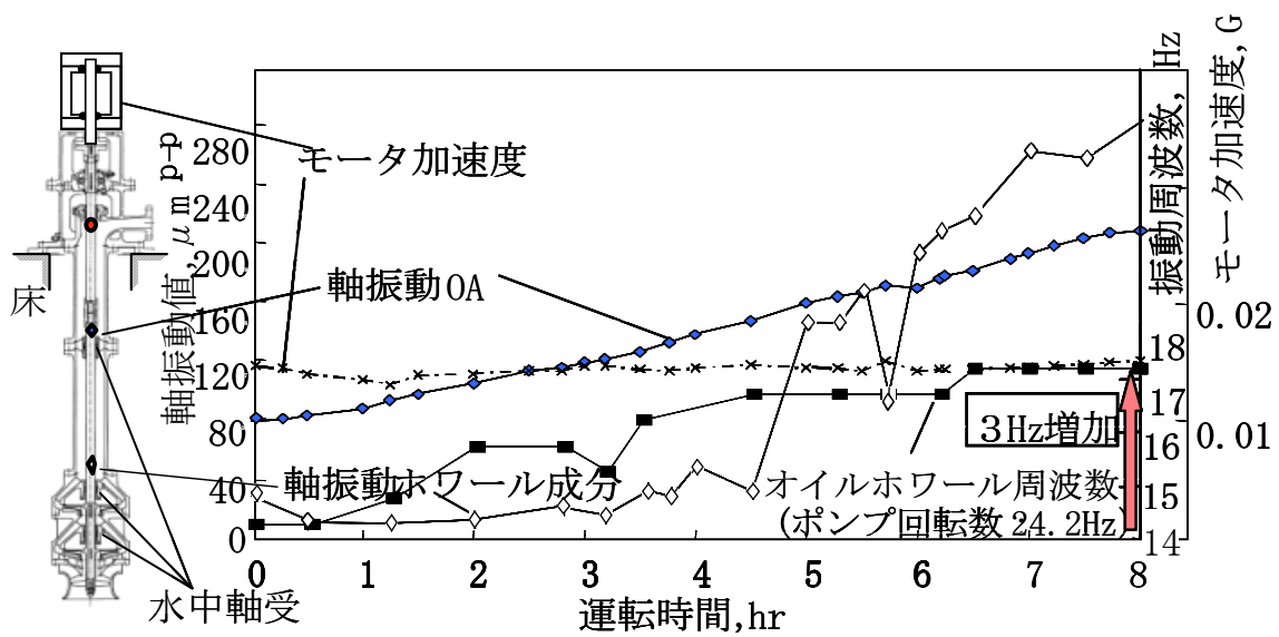
図 7.5.10 縦型ポンプの軸受摩耗加速試験
