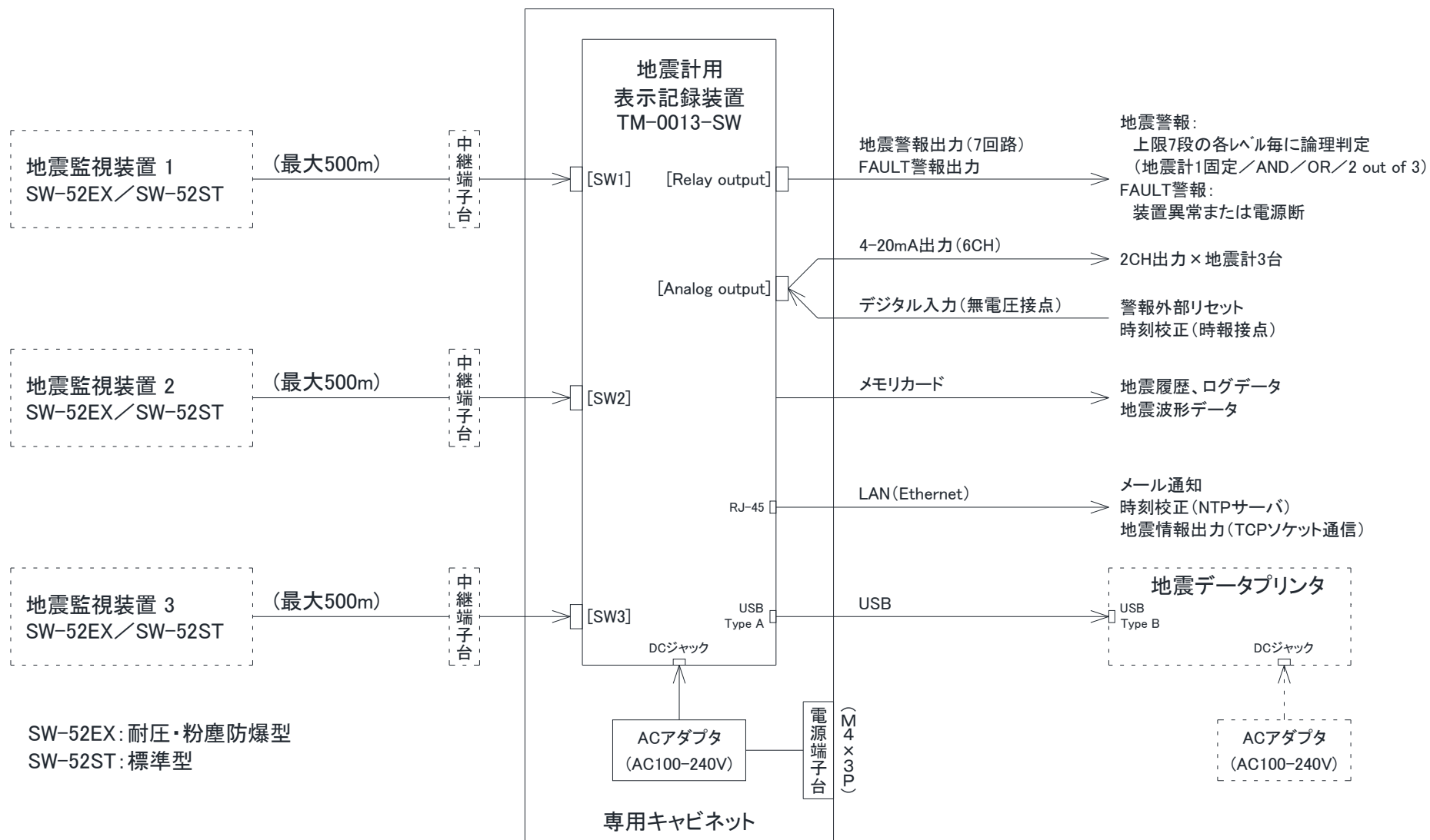
2-2. システム構成図
